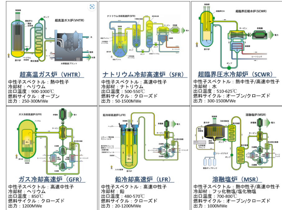
図2：GIFにおいて選定された第4世代原子炉システム
